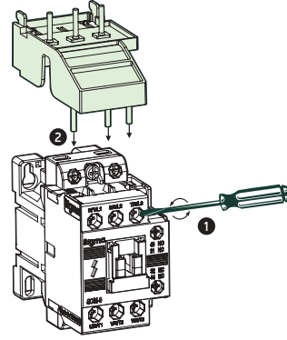
SMK25-A - Montaj
